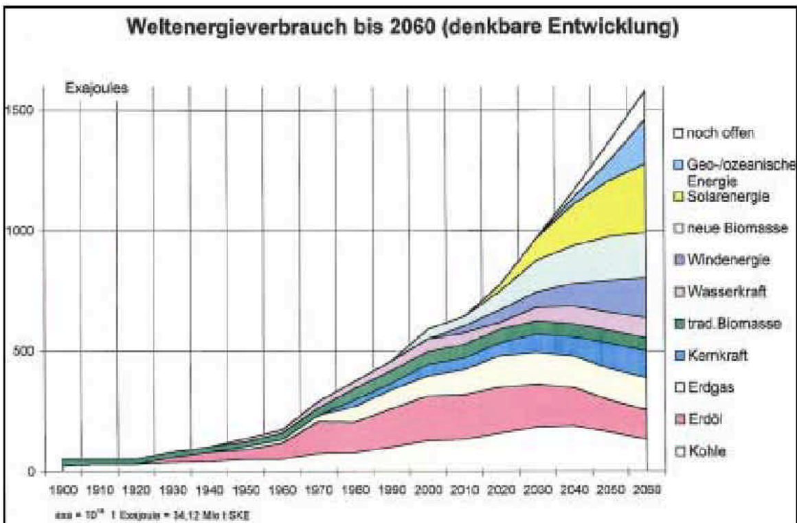
Abb. 2: Shell-Szenario zur Entwicklung des Weltenergieverbrauchs bis zum Jahre 2060
