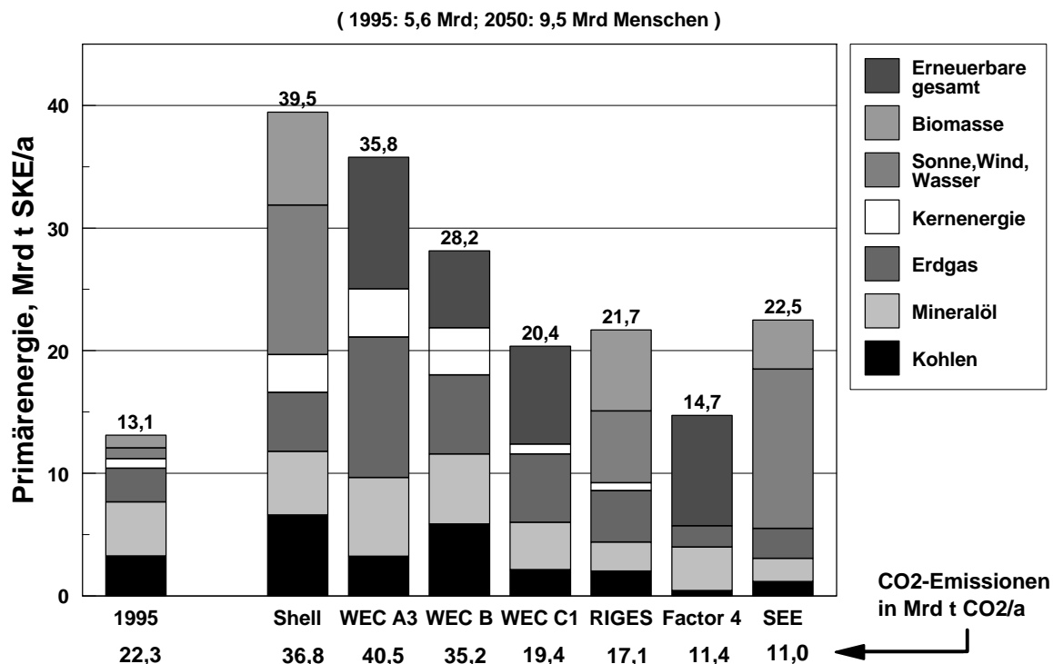
Abb. 1: Aktuelle Szenarien des Weltenergieverbrauchs für das Jahr 2050*
