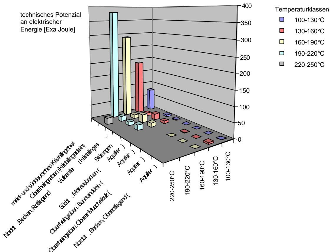
Abb. 18: Zusammenstellung der Verteilung des technischen Potenzials zur Stromerzeugung (ohne KWK-Betrieb) aller betrachteten Reservoirre nach Temperaturklassen
