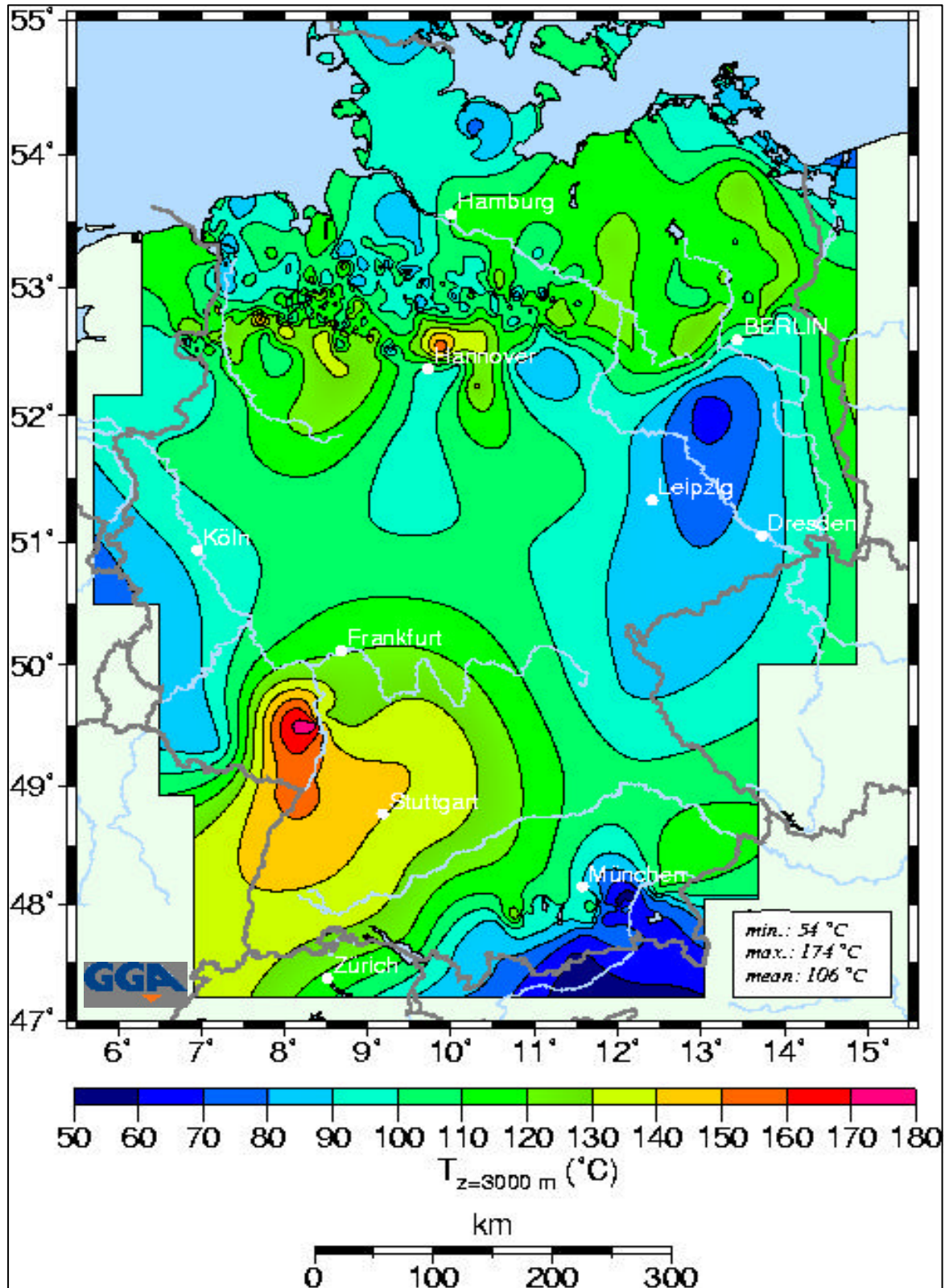
Abb. 2: Temperaturverteilung im Untergrund (ca. 3.000 m) in Deutschland
