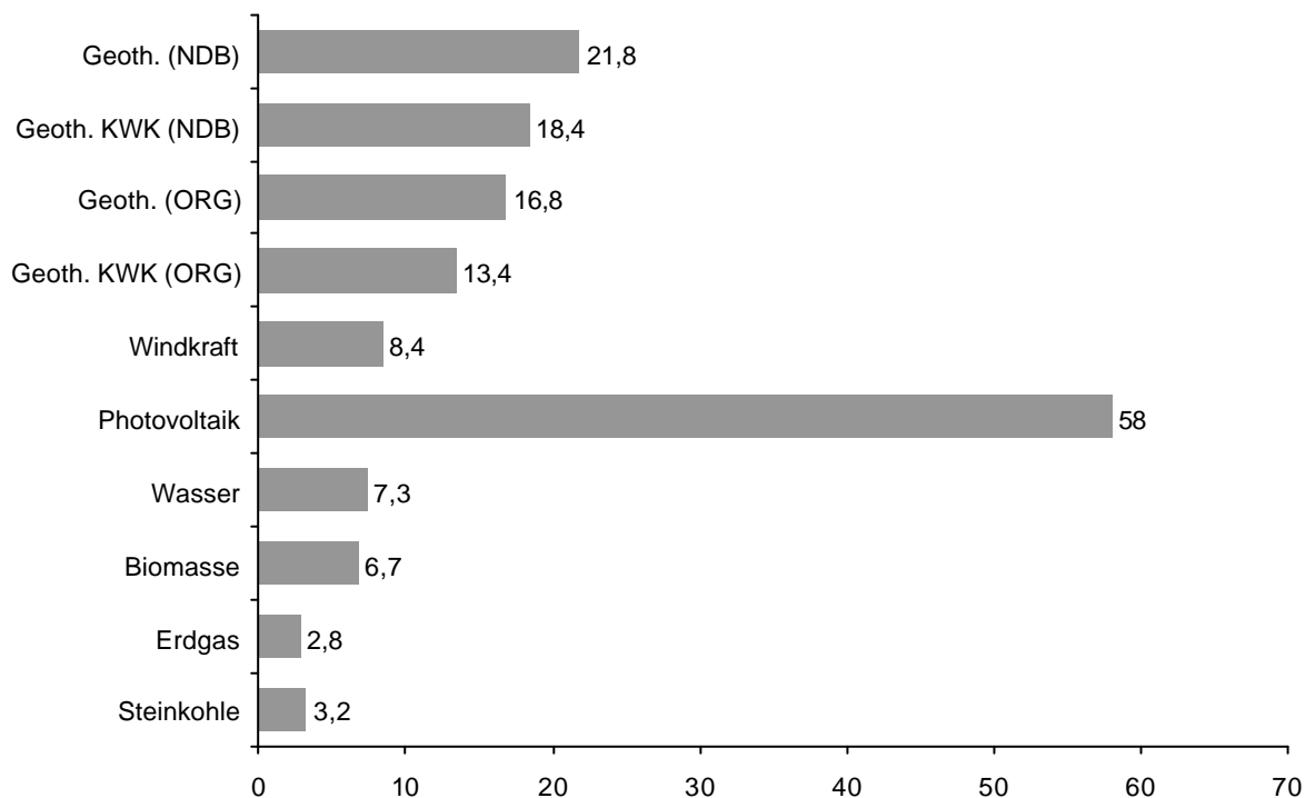
Abb. 24: Gestehungskosten einer Stromerzeugung aus regenerativen Energien, Erdgas, Steinkohle
