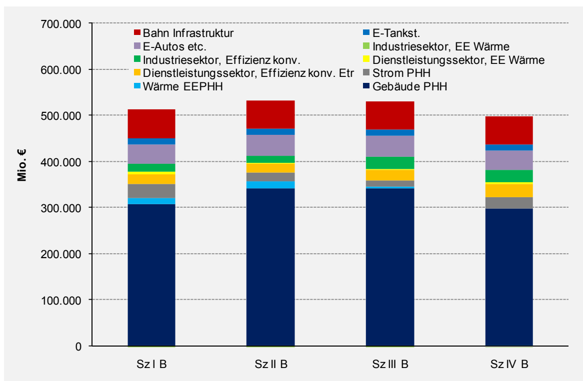
Abbildung 5.1.2.1-3: Kumulierte Investitionsdifferenzen in den Zielszenarien I B – IV B im Vergleich zur Referenz, in Mio EUR
