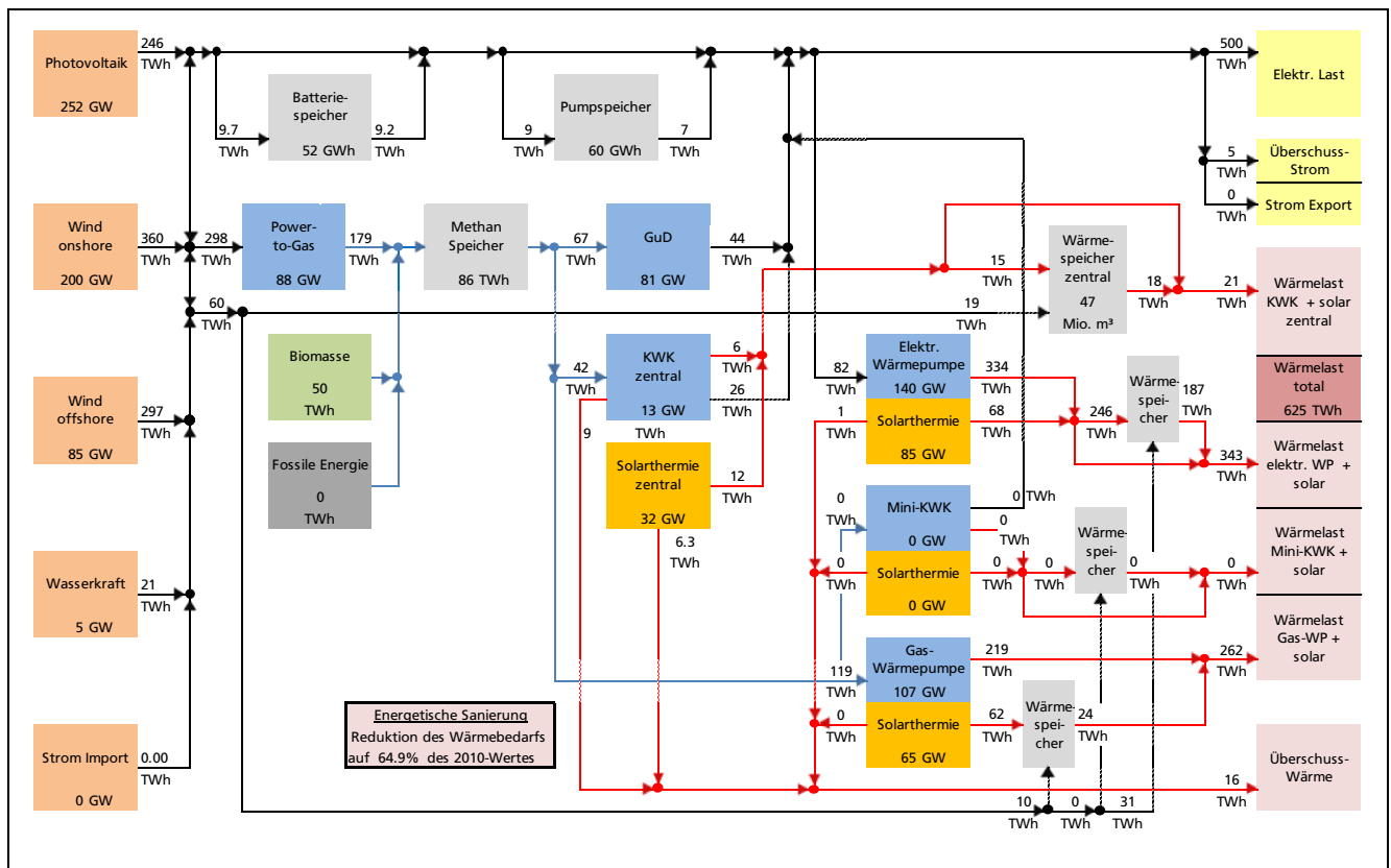
Abb. 6 System, das zu niedrigsten jährlichen Gesamtkosten führt
