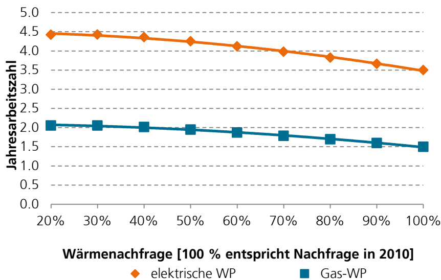
Abb. 4 Abhängigkeit der durchschnittlichen Jahresarbeitszahl der Wärmepumpen vom Sanierungszustand (oben: elektrische Wärmepumpe, unten: Gas-Wärmepumpe) (Quelle: Eigene Berechnung basierend auf Daten aus [20, 21])
