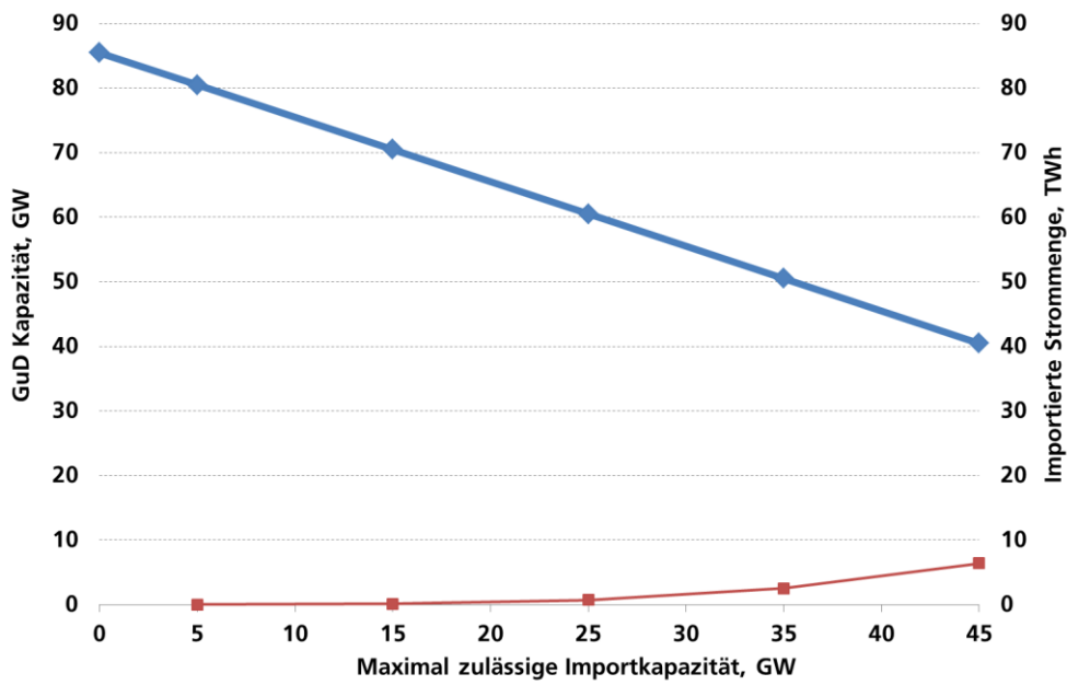
Abb. 14 Installierte GuD-Leistung und jährliche Importstrommenge in Abhängigkeit der maximalen Leistung von Stromimport
