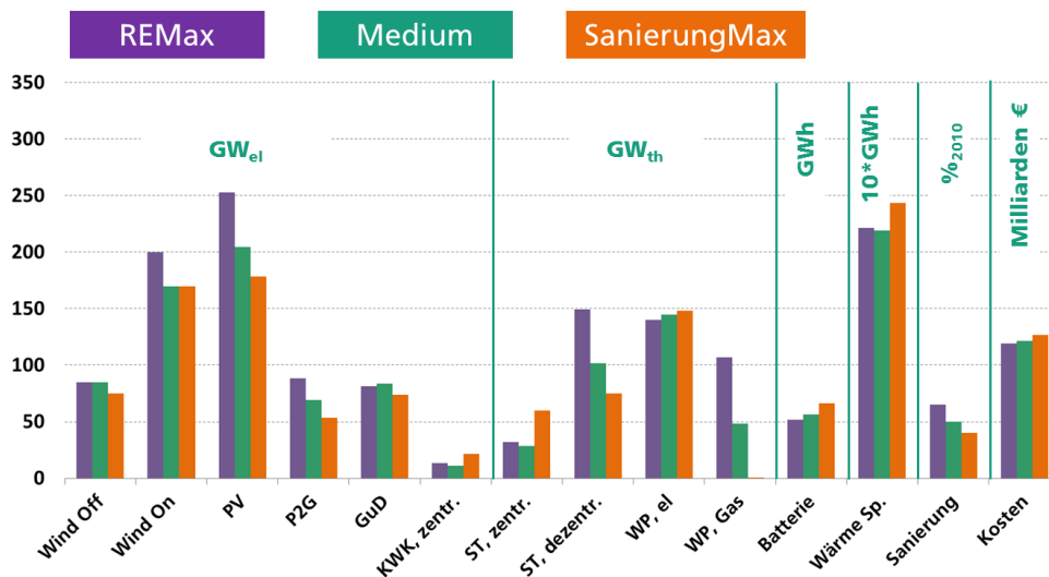
Abb. 8 Drei Systeme im Vergleich
