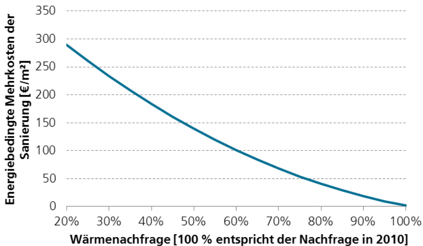
Abb. 3 Kostenverlauf der Energieeffizienz bedingten Mehrkosten für energetische Sanierung (in €/m 2 ) in Abhängigkeit des Grades der Energieeinsparung bezogen auf den Wert aus 2010 (Quelle: Eigene Berechnung basierend auf Daten aus [16-19])
