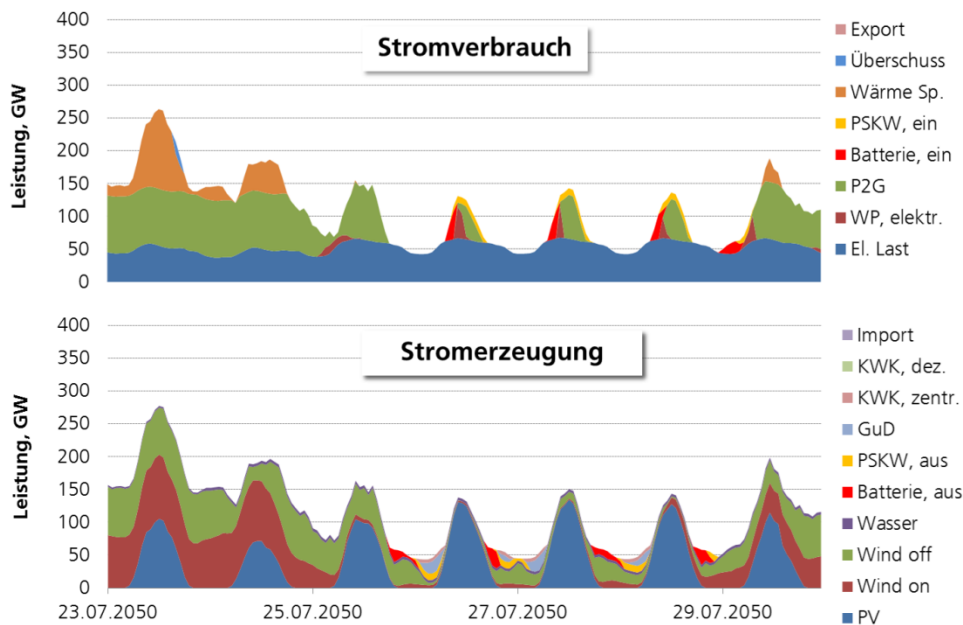
Abb. 11 Stromverbrauch und Stromerzeugung des Szenarios „Medium“ in einer Sommerwoche (PSKW=Pumpspeicherkraftwerk; P2G=Power-to-Gas; WP=Wärmepumpe; KWK=Kraft-Wärme-Kopplung).
