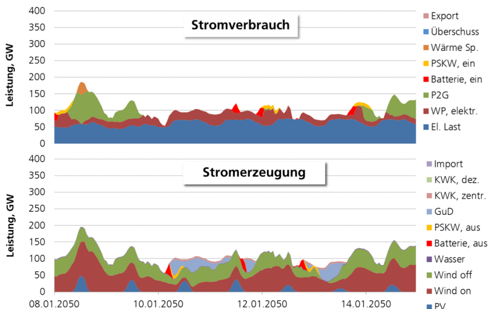
Abb. 9 Stromverbrauch und Stromerzeugung des Szenarios „Medium“ in einer Winterwoche (PSKW=Pumpspeicherkraftwerk; P2G=Power-to-Gas; WP=Wärmepumpe; KWK=Kraft-Wärme-Kopplung).
