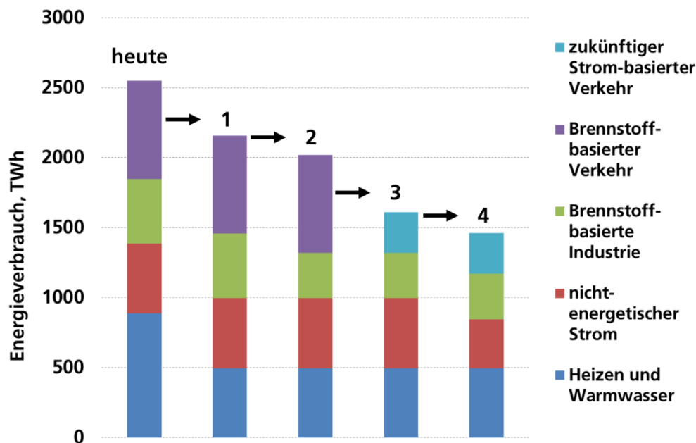
Abb. 15 Effizienz-Beiträge der verschiedenen Sektoren des Energieverbrauchs, um eine bilanzielle Deckung mit erneuerbaren Energien zu ermöglichen 1: Reduktion des Heizwärmebedarfs des Gebäudesektors um 50 % bezogen auf 2010 (wie in Kapitel 4 dargestellt) 2: Reduktion des Brennstoffverbrauchs in der Industrie um 30 % 3. Umstellung des heute Brennstoff-basierten Verkehrs auf Strom-basierten Verkehr (Annahme 50 % Batterie und 50 % Wasserstoff) 4. Reduktion des nicht-energetischen Stromverbrauchs um 30 % (Quelle: Eigene Darstellung)
