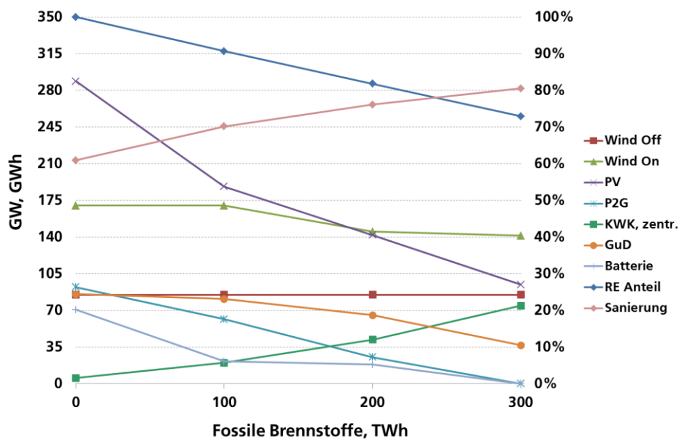
Abb. 13 Abhängigkeit der Größe zentraler Elemente des Energiesystems von der Menge verwendeter fossiler Brennstoffe
