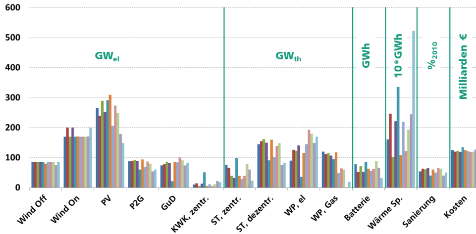
Abb. 7 unterschiedliche Systeme, die alle zu jährlichen Gesamtkosten im Bereich zwischen 119 Mrd. € und 126 Mrd. € führen
