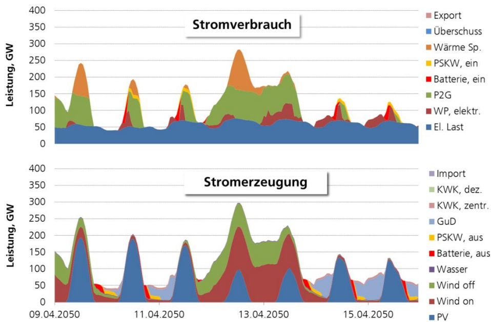
Abb. 10 Stromverbrauch und Stromerzeugung des Szenarios „Medium“ in einer Frühjahrswoche (PSKW=Pumpspeicherkraftwerk; P2G=Power-to-Gas; WP=Wärmepumpe; KWK=Kraft-Wärme-Kopplung).
