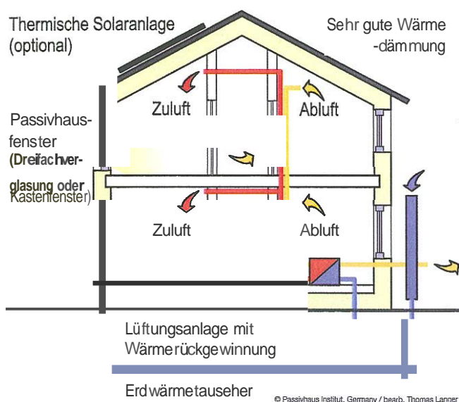
Schematische Darstellung eines Passivhauses
