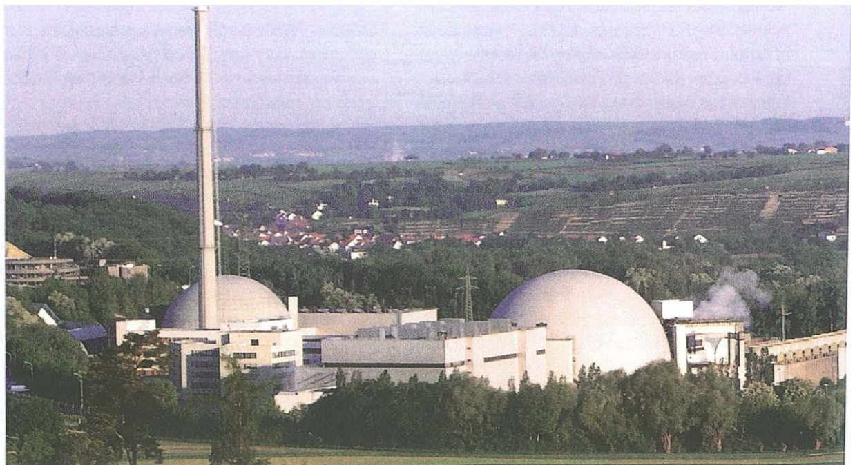
Kernkraftwerk Gemeinschaftskraftwerk Neckar (GKN) bei Neckarwestheim, aufgenommen vom Burgfried des Schloss Liebenstein. In der Bildmitte die Zellenkühler von Block 1, Rechts der Hybridkühlturm von Block 2. (Quelle: FZK)
