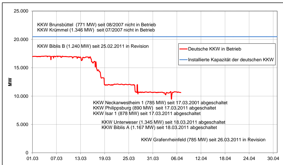
Abbildung 1 Installierte Leistung und Stromerzeugung der deutschen Kernkraftwerke, 2011
