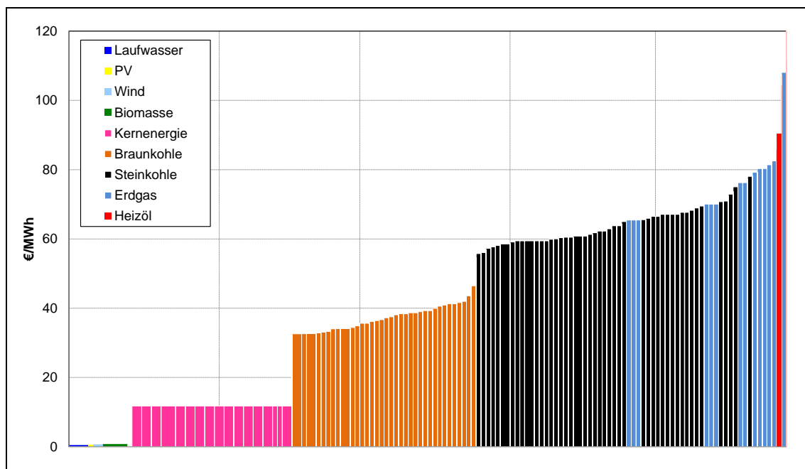
Abbildung 3 Schematische Darstellung der Merit-Oder und der Grenzkostenpreisbildung im liberalisierten Strommarkt
