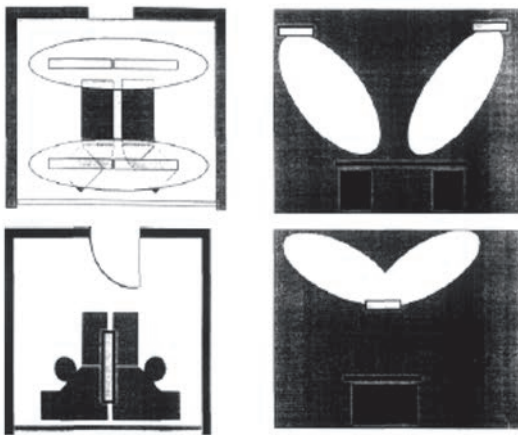
Рис. 2. Примеры расположения светильников: сверху – светильники с зеркальной решеткой 1 – 58 Вт, прямого света, четыре светильника справа и слева от рабочего места; снизу – светильники отраженного света 2 – 55 ватт висят непосредственно над рабочим местом
